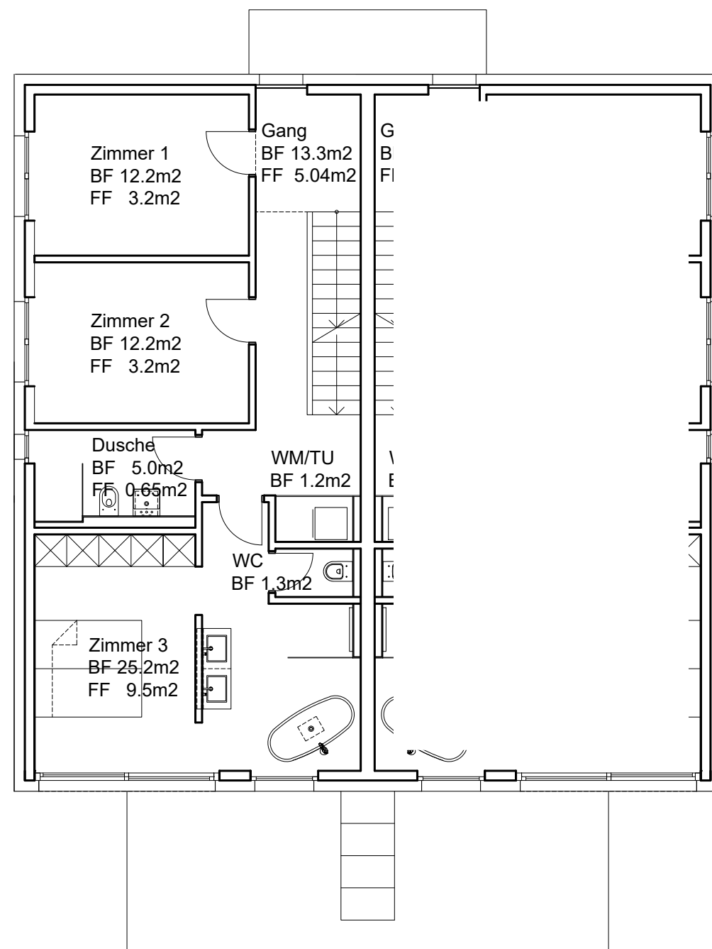
OBERGESCHOSS
